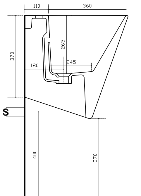
Sezione A-A Section A-A
