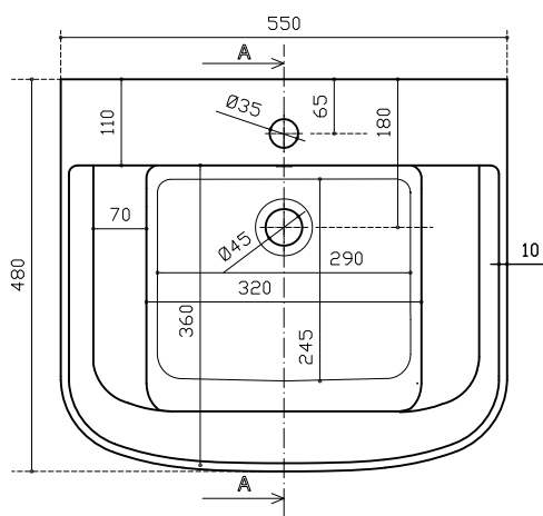
Vista dall'alto Top view
