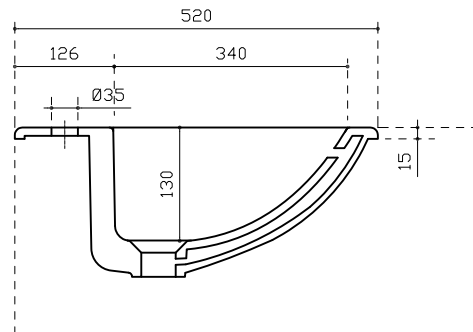
Vista laterale Lateral View Vista lateral Vue latérale
