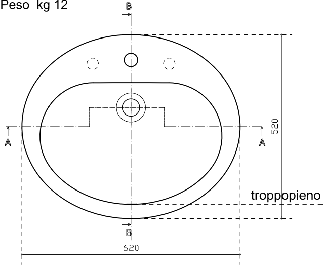
Vista dall'alto Top View Vista desde arriba Vue du haut
